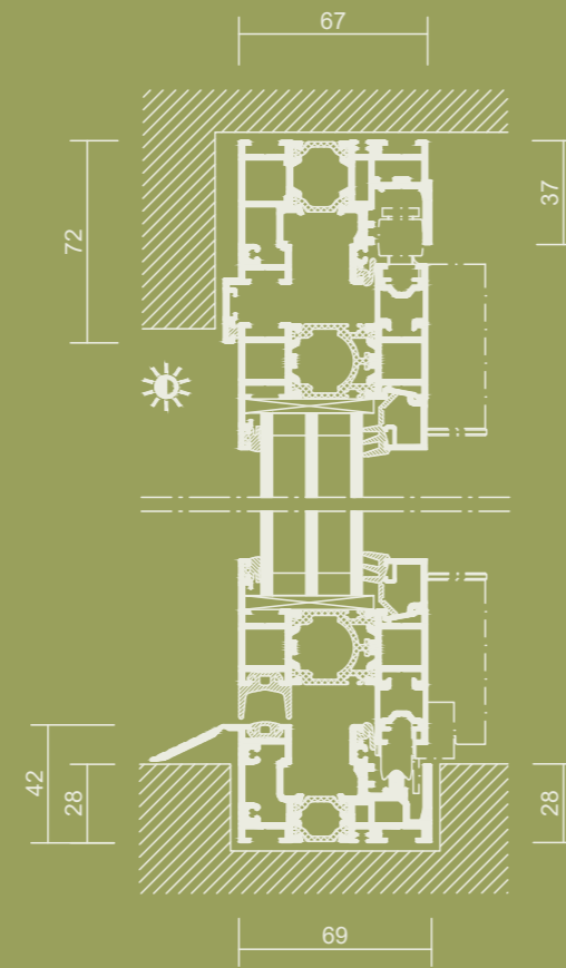
Vertikalschnitt | o.M.
