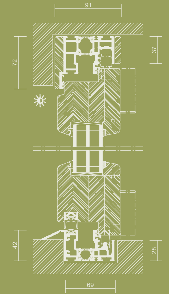
Vertikalschnitt | o.M.
